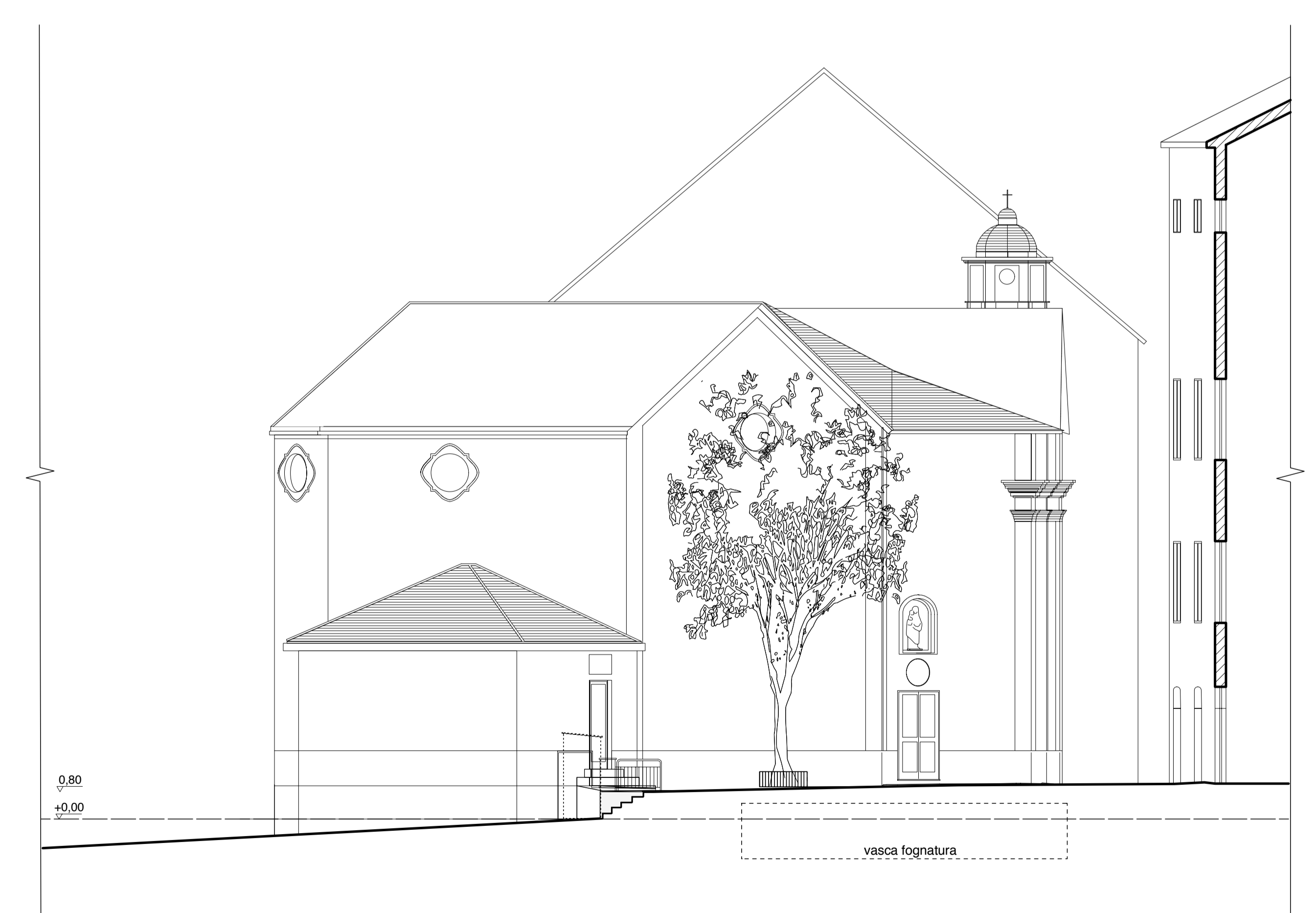
2 sezione AA scala 1: 100
